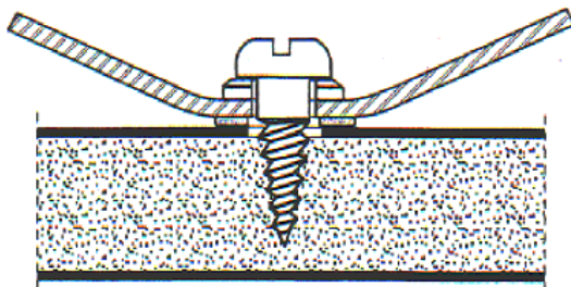
Abb.16: Verschraubung im Verbundelement
