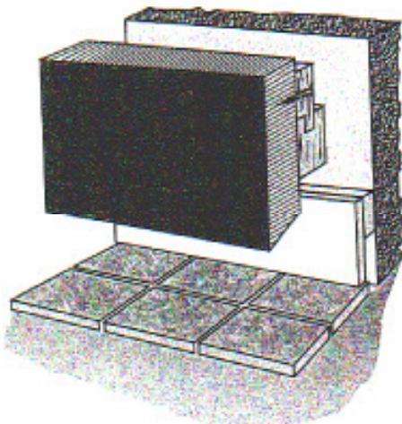
Abb. 4: Sockel aus Dekorativen Schichtstoffkompaktplatten
