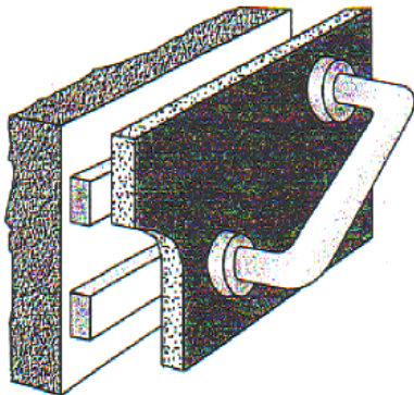
Abb.8: Verschrauben in der Unterkonstruktion
