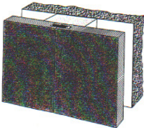
Abb. 6: Stumpfer Stoß mit Feder
