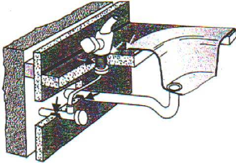
Abb. 15: Abdichtung von Durchführungen und Anschlüssen
