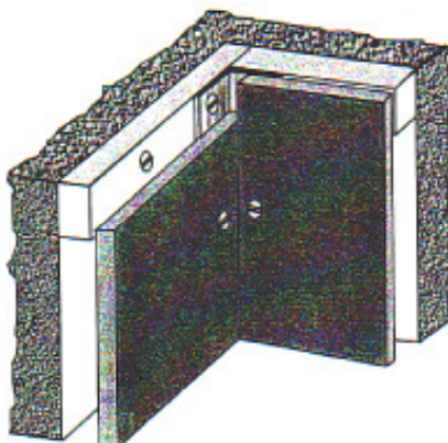
Abb. 8: Eckverbindung „Stumpfer Stoß“
