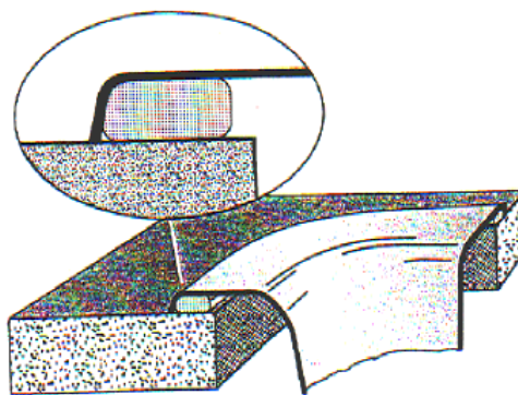
Abb. 14: Beckeneinbau mit verdeckter Trockendichtung
