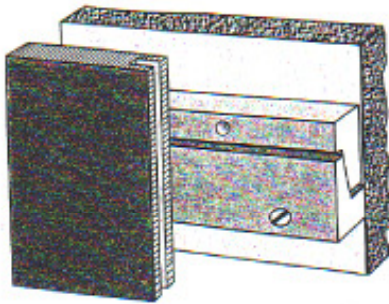
Abb.1: Befestigungsart „Einhängen“
