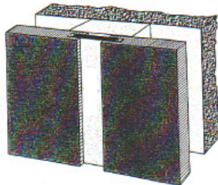
Abb. 7: Schattenfuge
