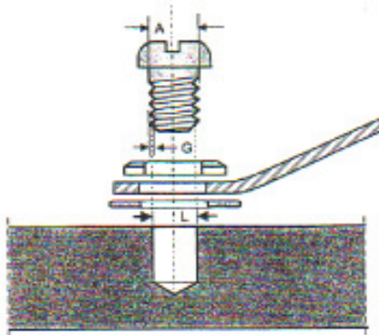
Abb.17: Verschraubung in Dekorativen Schichtstoffkompaktplatten
