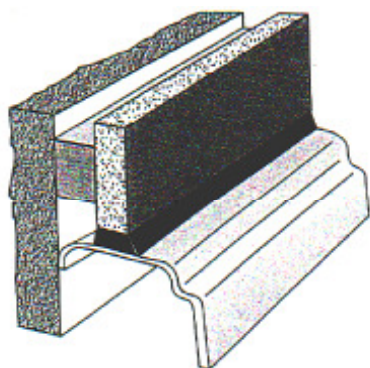
Abb. 13: Wannenanschluss mit dauerelastischer Dichtungsmasse
