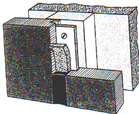
Abb.11: Fuge mit Dichtungsmasse
