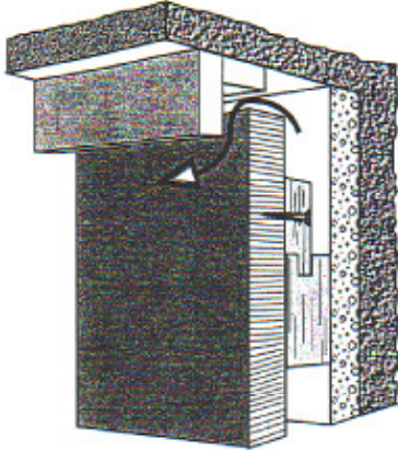
Abb. 5: Passblende für Raumüberhöhen, Deckenanschluss mit Blende
