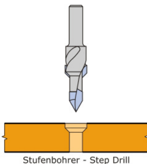
Abbildung 15: Absatz- / Stufenbohrer (Quelle: Leitz GmbH & Co. KG)
