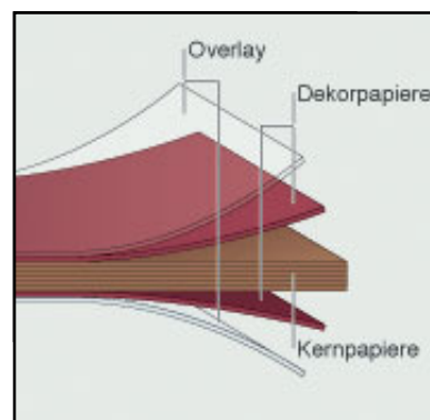
Abbildung 2: Kompaktplatte
