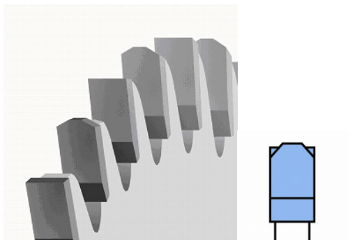
Abbildung 10: Trapezzahn / Flachzahn (Quelle: Leitz GmbH & Co. KG)
