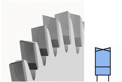
Abbildung 9: Wechselzahn (Quelle: Leitz GmbH & Co. KG)
