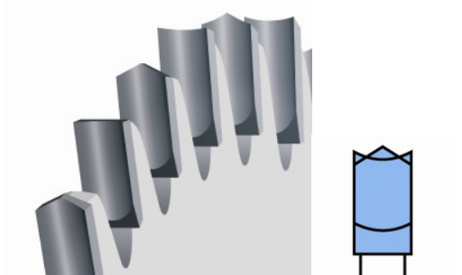
Abbildung 11: Dachzahn / Hohlzahn (Quelle: Leitz GmbH & Co. KG)
