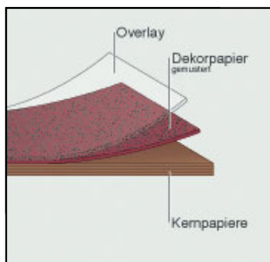
Abbildung 1: Schichtstoffplatte
