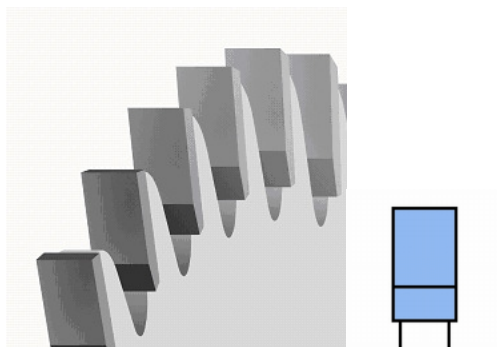
Abbildung 8: Flachzahn (Quelle: Leitz GmbH & Co. KG)
